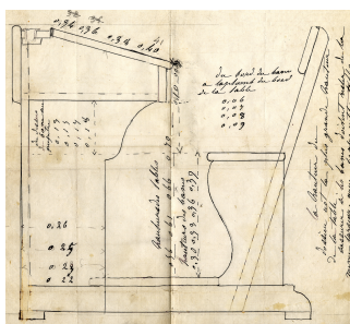
Coupe latérale de la table-banc des écoles du Familistère. Dessin de Jean-Baptiste André Godin, janvier 1873. Collection archives départementales de l'Aisne. Crédit photographique : archives départementales de l'Aisne.
